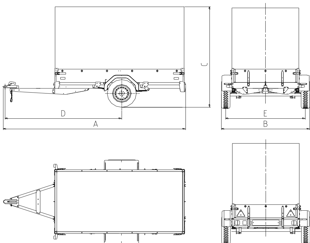
Рис. 2 – Общий вид одноосного прицепа с бортовой платформой или фургонем (ССТ-7132-01, ССТ-7132-02, ССТ-7132-03, ССТ-7132-06, ССТ-7132-08, ССТ-7132-09)
