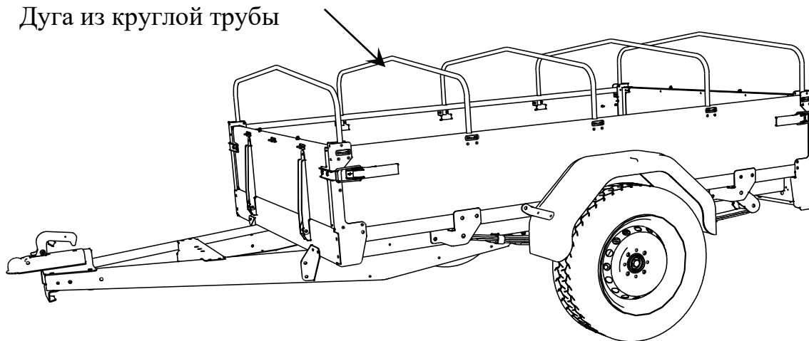
Схема установки надставных бортов
