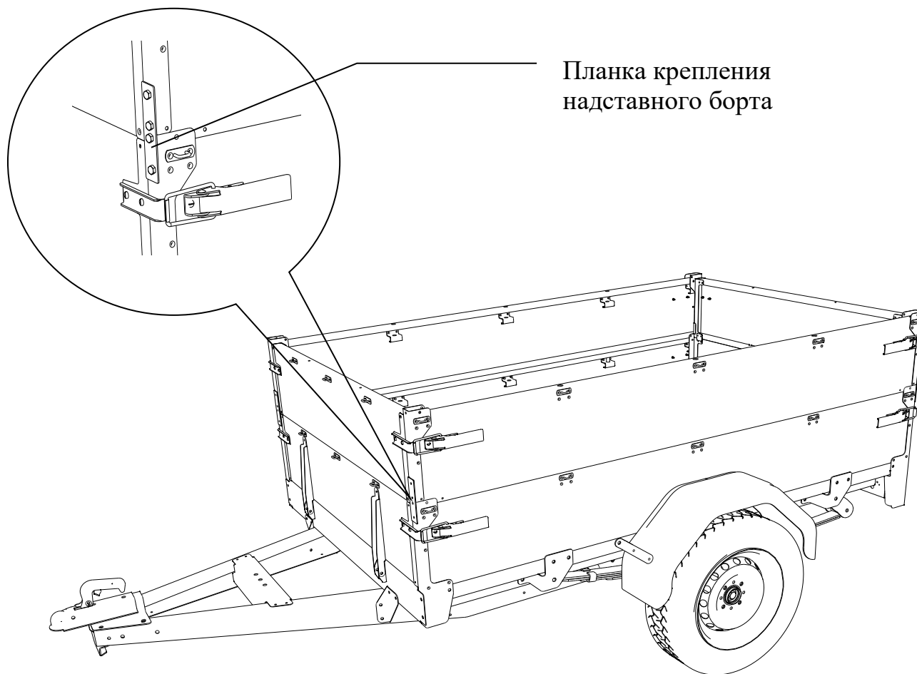
Схема установки надставных бортов
